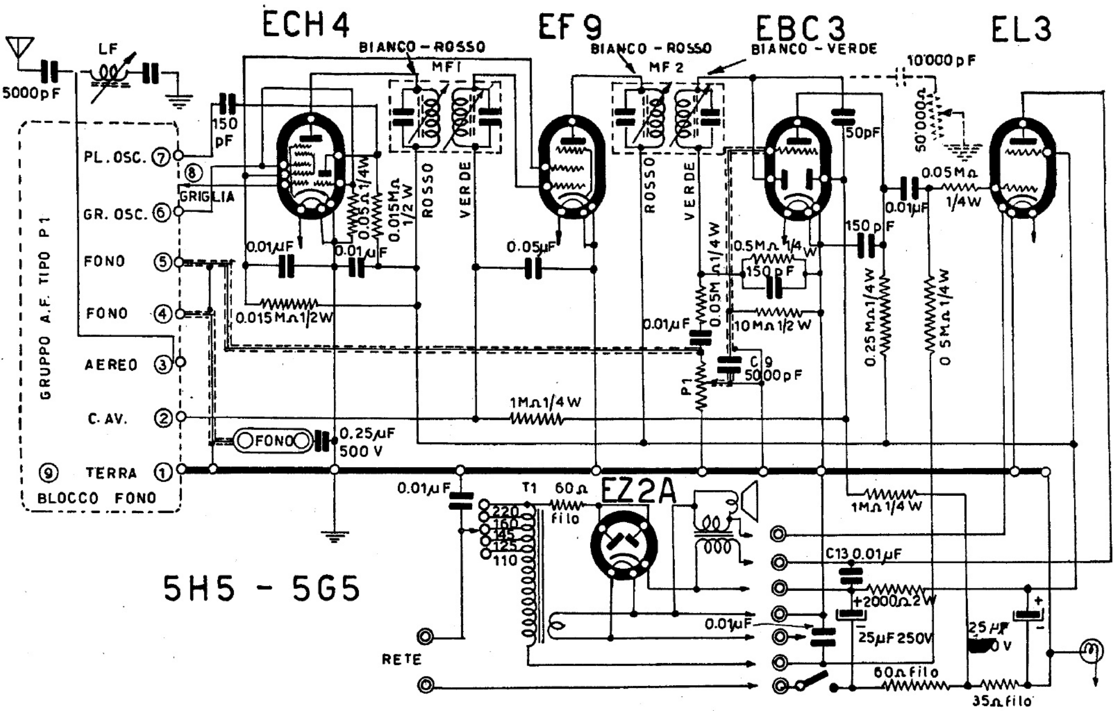
NOVA RADIO - Mod. 5G5 e mod. 5H5. Gamma onde medie divisa, tre gamme onde corte. Media frequenza 465 kc/s. (V. a parte lo schema del gruppo AF P1). Il controllo di tono (parte tratteggiata) è presente solo nel mod. 5H5.
